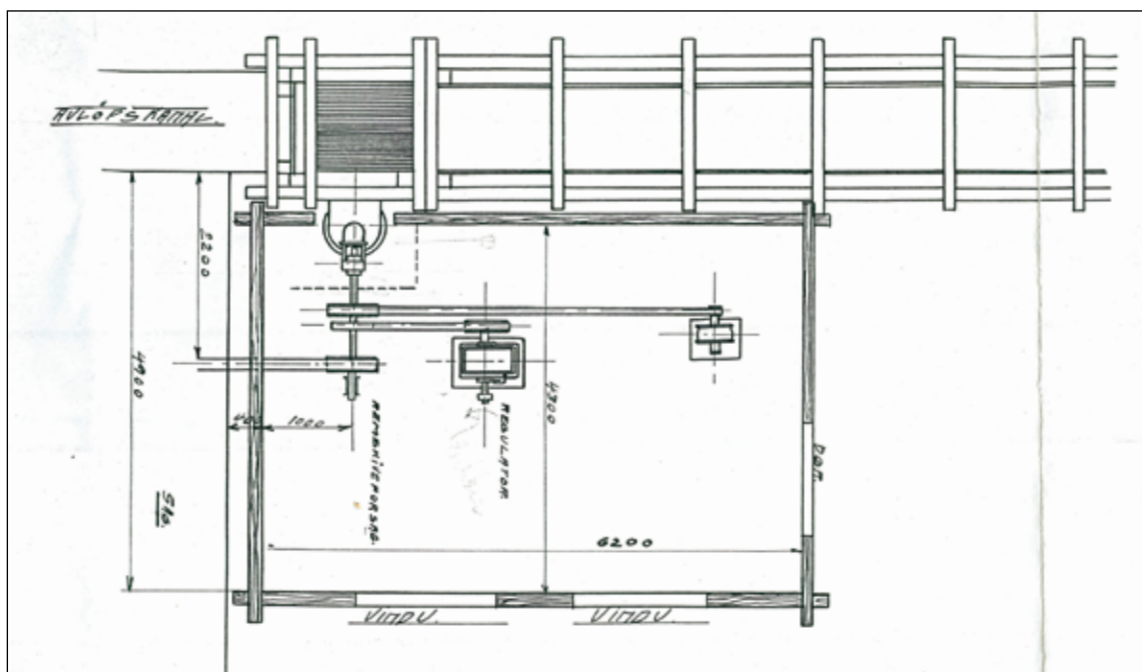
Innvendig i Nylendfossen kraftstasjon. Vannet kom i renne/rør utenfor huset og rant gjennom turbinen. Kraften fra turbinen ble overført via remmer til en generator.
