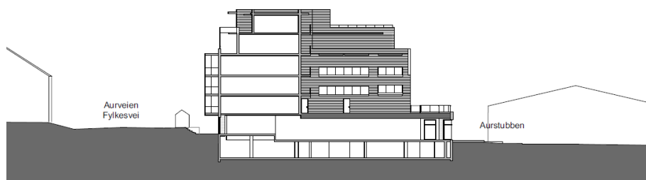
Tverrsnitt av bygg E i enden av kvartalet
