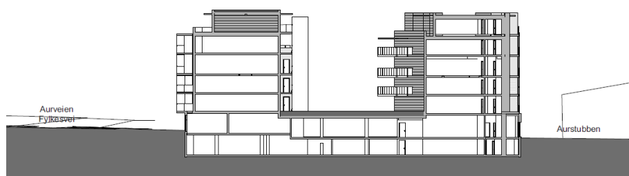
Tverrsnitt gjennom bygg C og D i midtre del av kvartalet.
